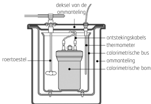
Fig. 8. Bomcalorimeter (NBN EN ISO 1716)
